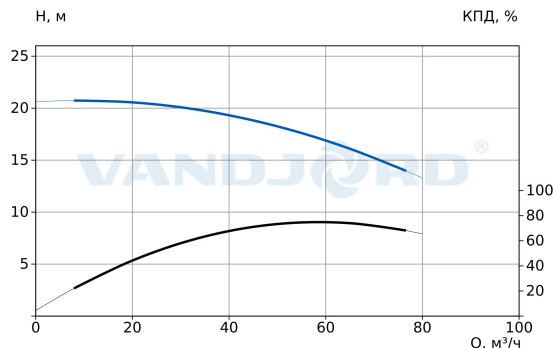
73116131 TPV 80-170-4/2 Q-A-BT-E
