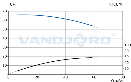
73114126 TPV 50-580-15/2 Q-A-BT-E
