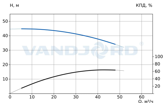
73114124 TPV 50-390-7.5/2 Q-A-BT-E
