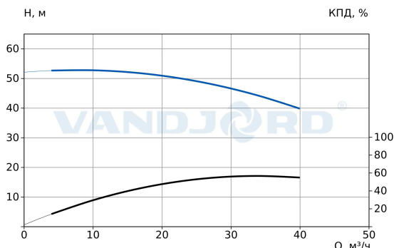
73113118 TPV 40-430-7.5/2 Q-A-BT-E
