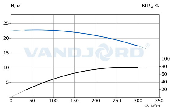
73119104 TPV 150-190-18.5/4 Q-A-B-E
