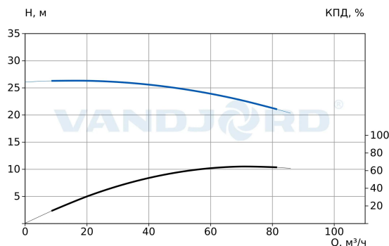
73116128 TPV 80-230-7.5/4 Q-A-B-E
