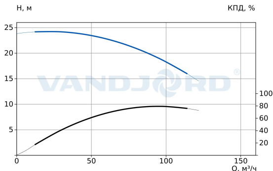
73117103 TPV 100-200-7.5/2 Q-A-B-E
