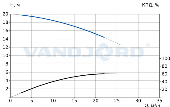
73114102 TPV 50-170-1.5/2 Q-A-B-E
