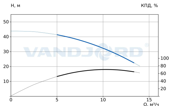
74137020 CRV 10-4CN A-D-E-HQQE-E
