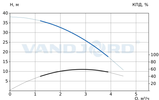
74113748 CRV 3-6C A-D-E-HQQE-E
